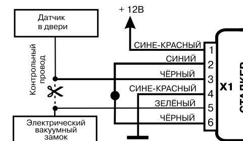
Рис. 7. Схема подключения к вакуумному центральному замку
