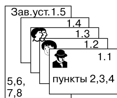
Рис. 18. Структура таблицы программирования Если программируются пункты 2,3,4, то не забудьте войти в нужную таблицу пользователя (1.1, 1.2, 1.3 или 1.4). Установка п. 1.5 сбросит ВСЕ эти таблицы в заводские установки (отмечены знаком *)
