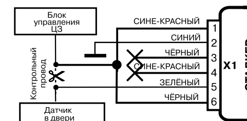
Рис. 8. Схема подключения к центральному замку, которому для отпирания требуется отрицательный импульс, а для запирания - разьединения проводов
