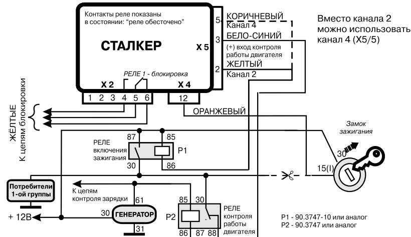
Рис. 14. Цепи для реализации режима "турбо"
