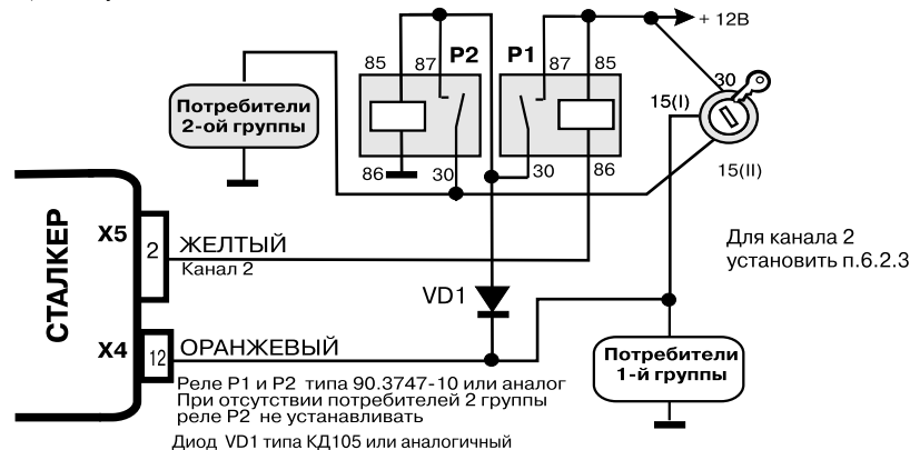
Рис. 15. Схема подачи зажигания при постановке на охрану с заведённым двигателем без ключа в замке зажигания
