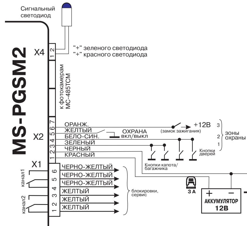
Рис.3. Подключение MS-PGSM2 в качестве охранной сигнализации.
