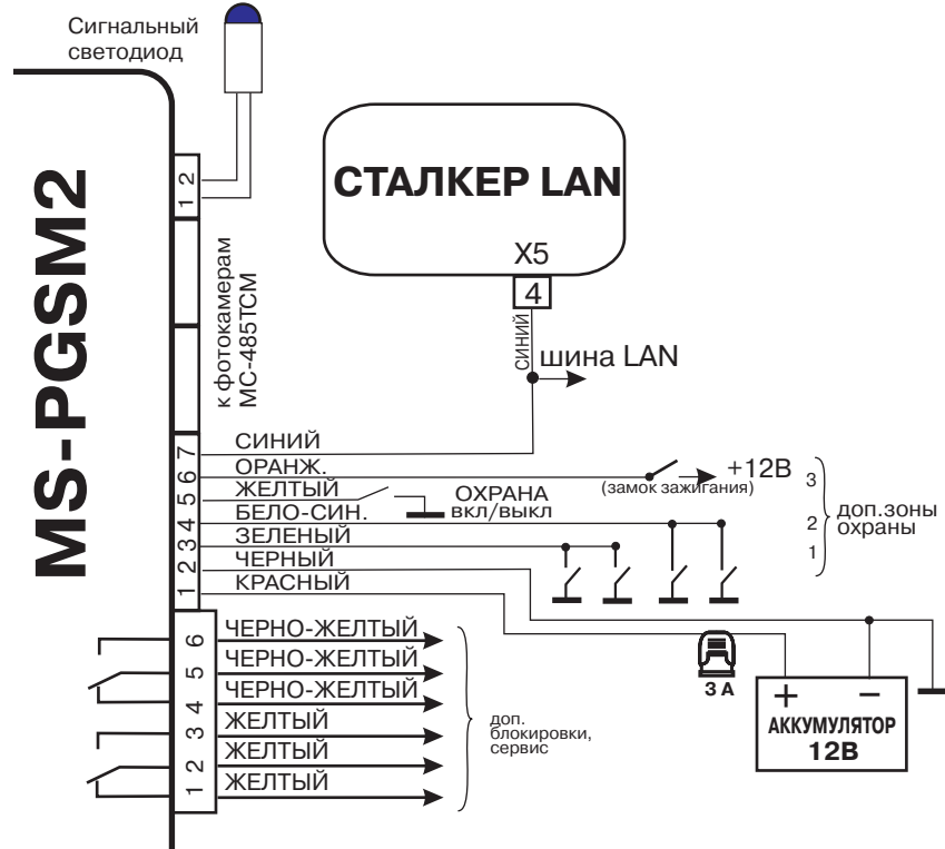
Рис.2. Подключение MS-PGSM2 по шине LAN к охранному комплексу СТАЛКЕР LAN 2
