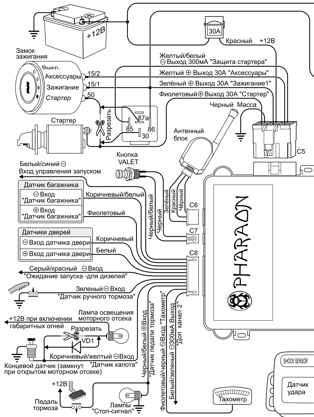
Рис. 1. СХЕМА ПОДКЛЮЧЕНИЯ PHARAO V20
