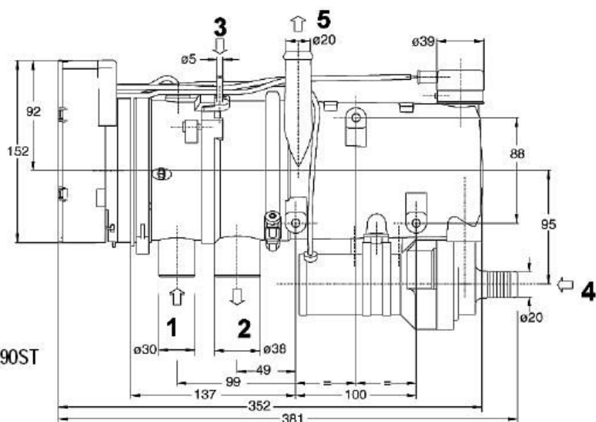
Рис. 2 Габариты подогревателя
