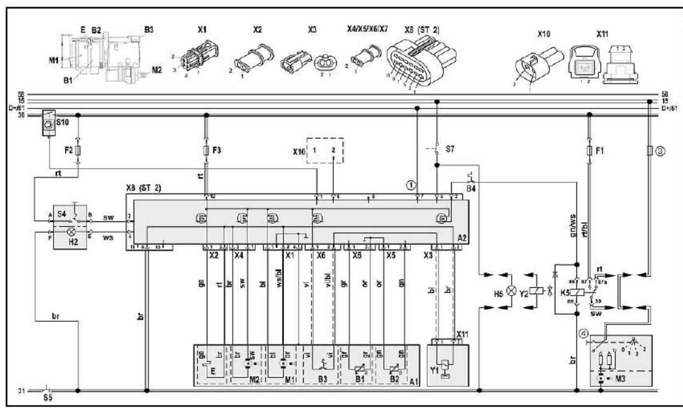
Рис. 20 Электросхема Thermo 90ST, 12 и 24 В, со стандартным таймером и сепаратно управляемым циркуляционным насосом, легенду см. стр. 16
