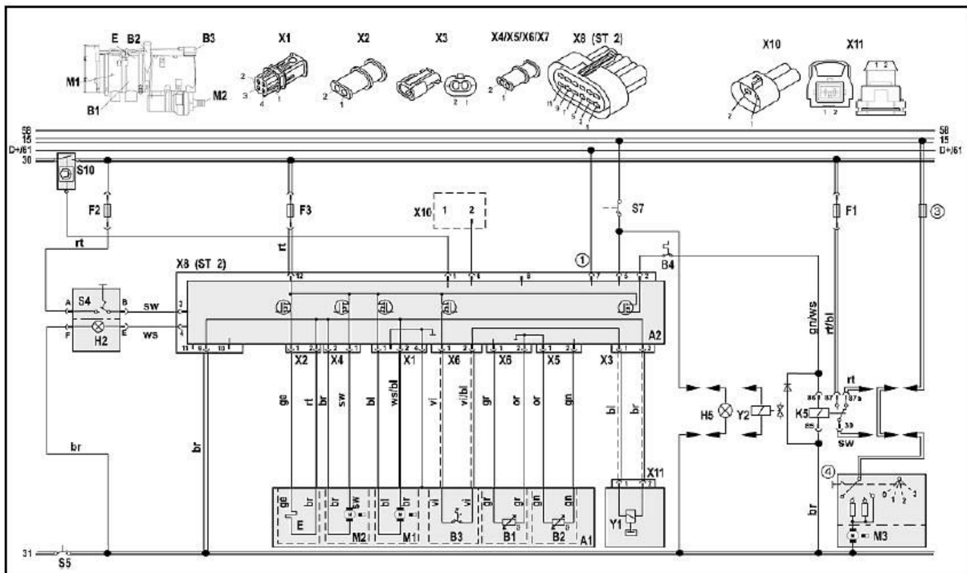
Рис. 21 Электросхема Thermo 90ST, 24 В, с выключателем, легенду см. стр. 16 (показан вариант подключения в автомобилях, перевозящих опасные грузы)
