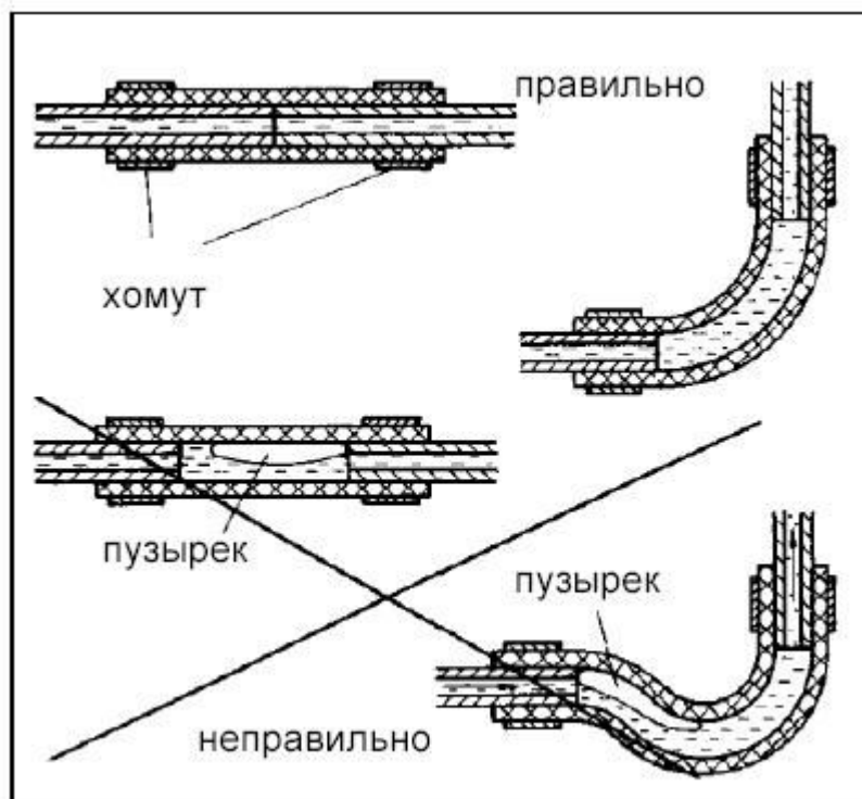
Рис. 4 Соединение трубы/шланги
