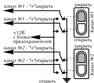
B_1 Кнопки с положительными сигналами при нажатии.
