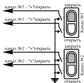
B_3 Вариант подключения кнопок на замыкание.
