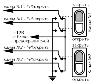
B_2 Кнопки с отрицательными сигналами при нажатии.
