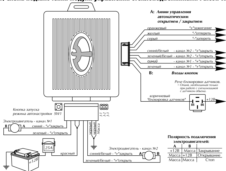
Рис. 1. Схема подключения модуля управления стеклоподъемниками Falcon WR-250
