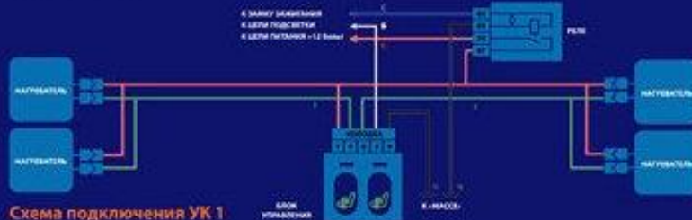
Схема подключения УК 1
