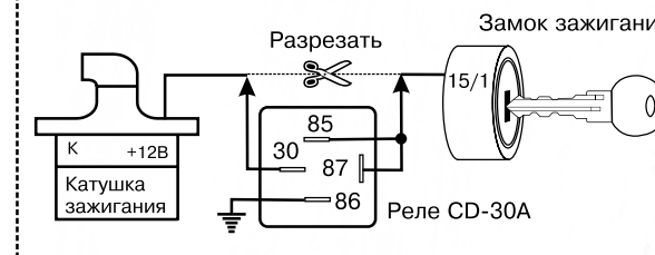
Схема блокировки зажигания посредством дистанционно управляемого реле CD-30A (Входит в комплект).
