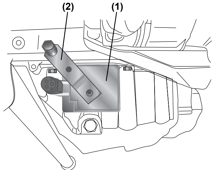
Пример контактного нагревателя (1), установленного на масляном картере и закрепленного держателем (2).
